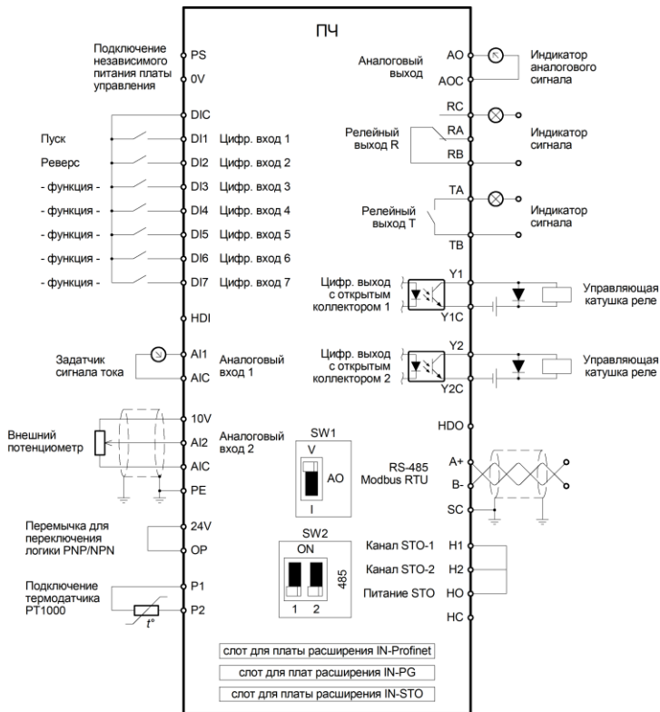
Рисунок 4 – Подключение управляющих клемм для преобразователя частоты серии INPRIME (плата IN-I/O-A)
