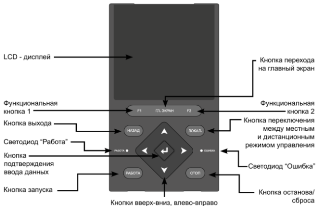
Рисунок 5 – Описание панели управления INPRIME
