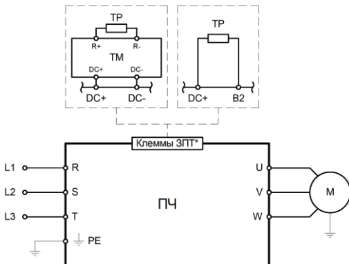
Рисунок 2 – Подключение силовых клемм для преобразователя частоты серии INPRIME до 75 кВт
