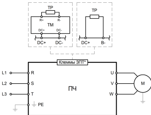
Рисунок 3 – Подключение силовых клемм для преобразователя частоты серии INPRIME от 90 кВт
